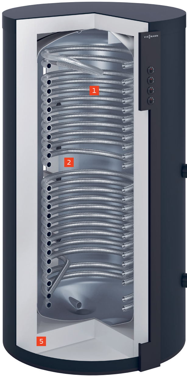
VITOCCELL 320-M dargestellt Typ SVHA (750 l) 1 Edelstahl-Wellrohr zur Trinkwasser- erwärmung 2 Speicherbehälter 3 Anschluss Elektro-Heizeinsatz (Zubehör) für die Komfortfunktion im Sommerbetrieb 4 Anschluss Elektro-Heizeinsatz (Zubehör) für die Einbindung von Photovoltaik-Anlagen 5 Abnehmbare Wärmedämmung
