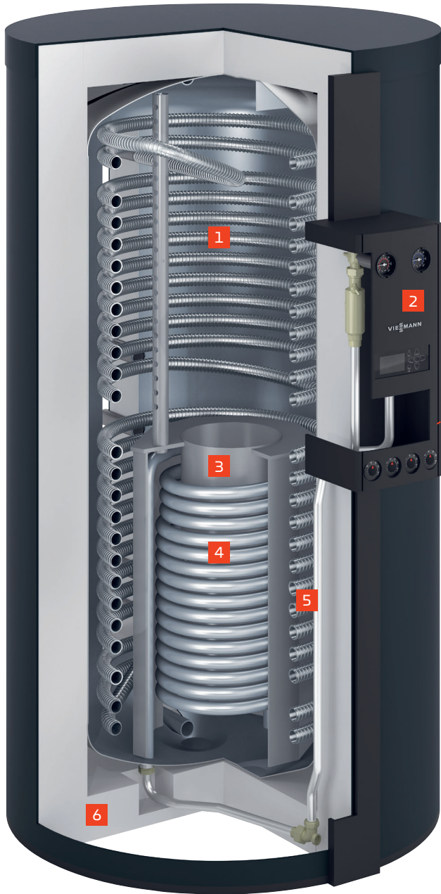
VITOCELL 360-M dargestellt Typ SVSB-750-S1 (750 l) mit Solar-Divicon (Zubehör)
