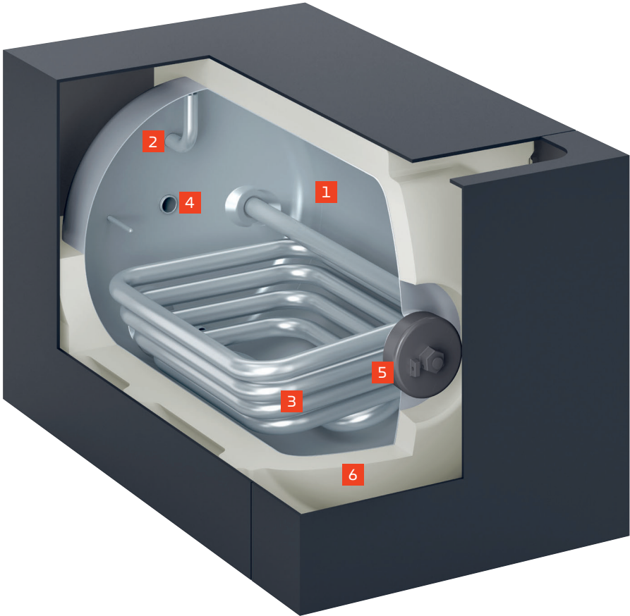
VITOCELL 300-H dargestellt Typ EHAA (160 l)
