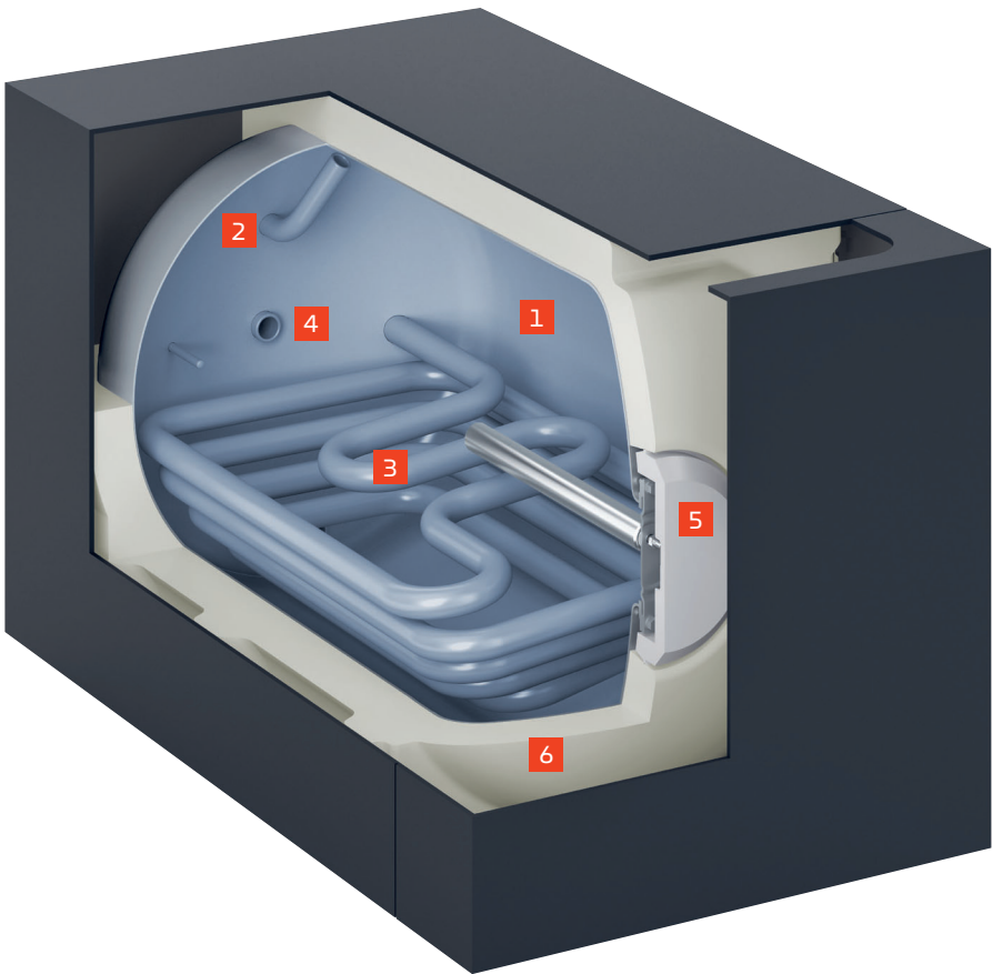
VITOCCELL 100-H dargestellt Typ CHAA (160 l)
