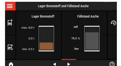
Ecotronic Touch - Anzeige Brennstofflager und Aschefüllstand
